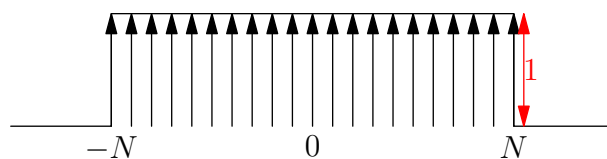
Σχήμα 6: Οι συντελεστές Fourier του πυρήνα του Dirichlet D_N(x) για N = 10
