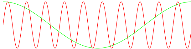
Σχήμα 1: Μια συνάρτηση που είναι “πιο συνεχής” από μια άλλη
