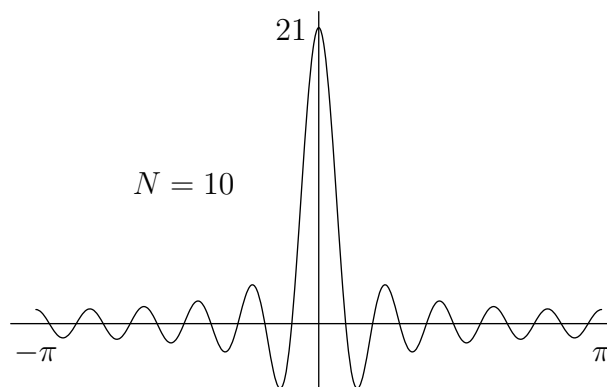
Σχήμα 5: Ο πυρήνας του Dirichlet
