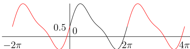
Σχήμα 2: Η διαδικασία της επέκτασης μιας συνάρτησης σε περιοδική (περιοδικοποίηση). Το γράφημα στα διαστήματα [-2\pi, 0] και [2\pi, 4\pi] είναι μεταφορές του γραφήματος στο διάστημα [0, 2\pi]
