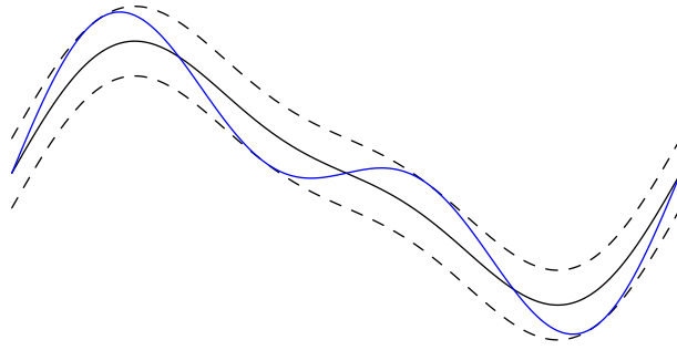
Σχήμα 3: Η βέλτιστη πολυωνυμική προσέγγιση (μπλε) της συνάρτησης πρέπει να ακουμπάει και το σύνορο της \rho -ζώνης (διακεκομμένη γραμμή) και προς τα πάνω και προς τα κάτω. Εδώ \rho = \|f - p^*\|_\infty .
